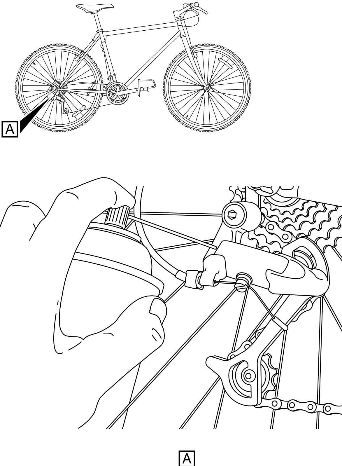
Fig 1 Derailleur pivots
