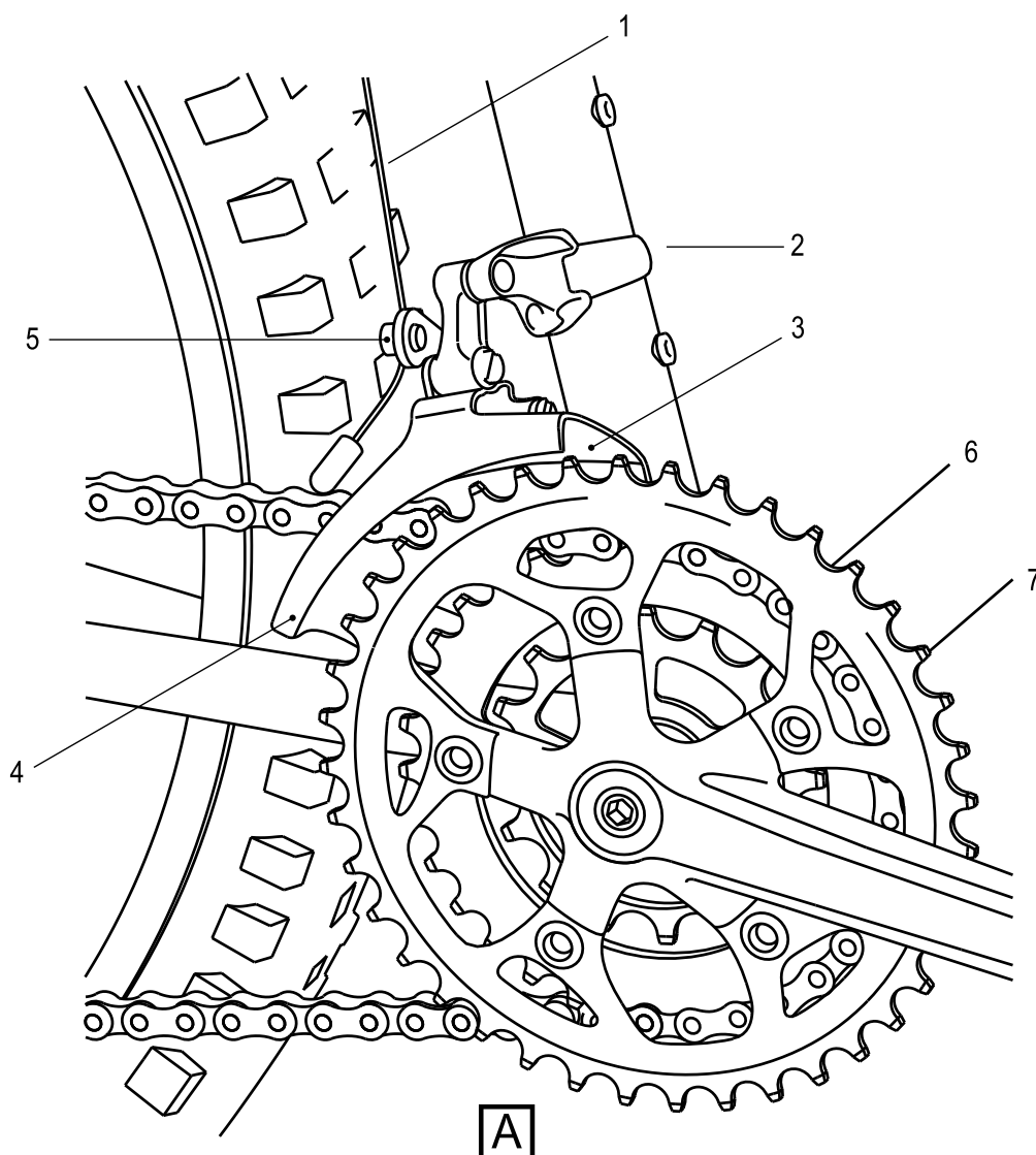
Fig 1 Front derailleur
